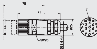
LTS.7 Grindbryter med nødstop + 10m kabel. Cat4/PLe, IP65.
